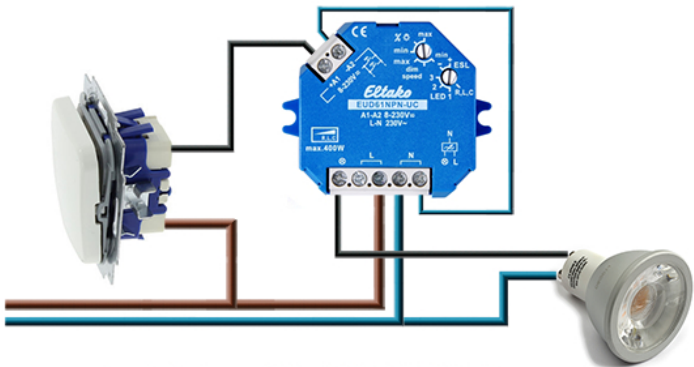
Aansluitschema Ellako EUD61NPN-UC dimmer
